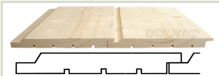
Profilis LN - lygus paviršius; LNS - šiurkštus paviršius
