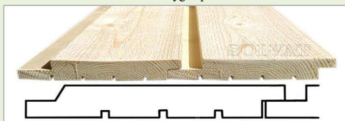
Profilis LE - lygus paviršius; LES - šiurkštus paviršius
